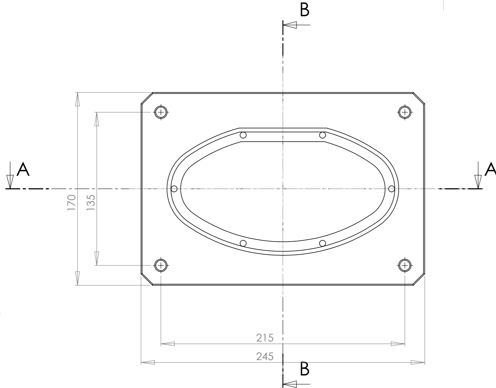
ŘEZ A-A
